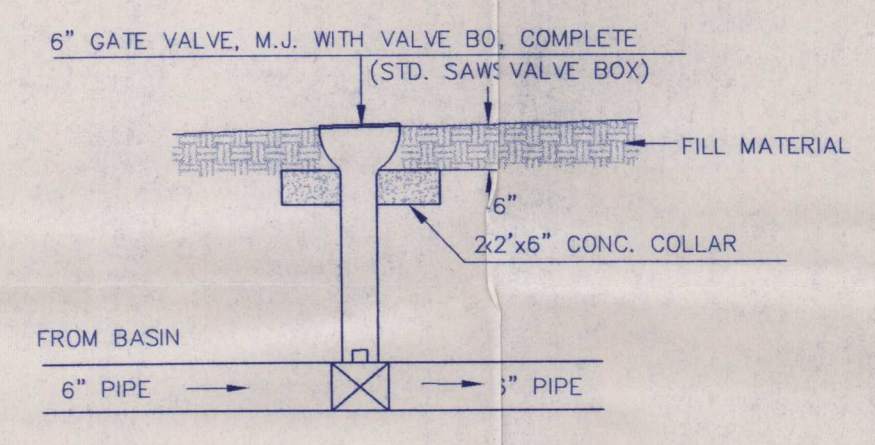
6 INCH GATE VALVE DETAIL N.T.S.
